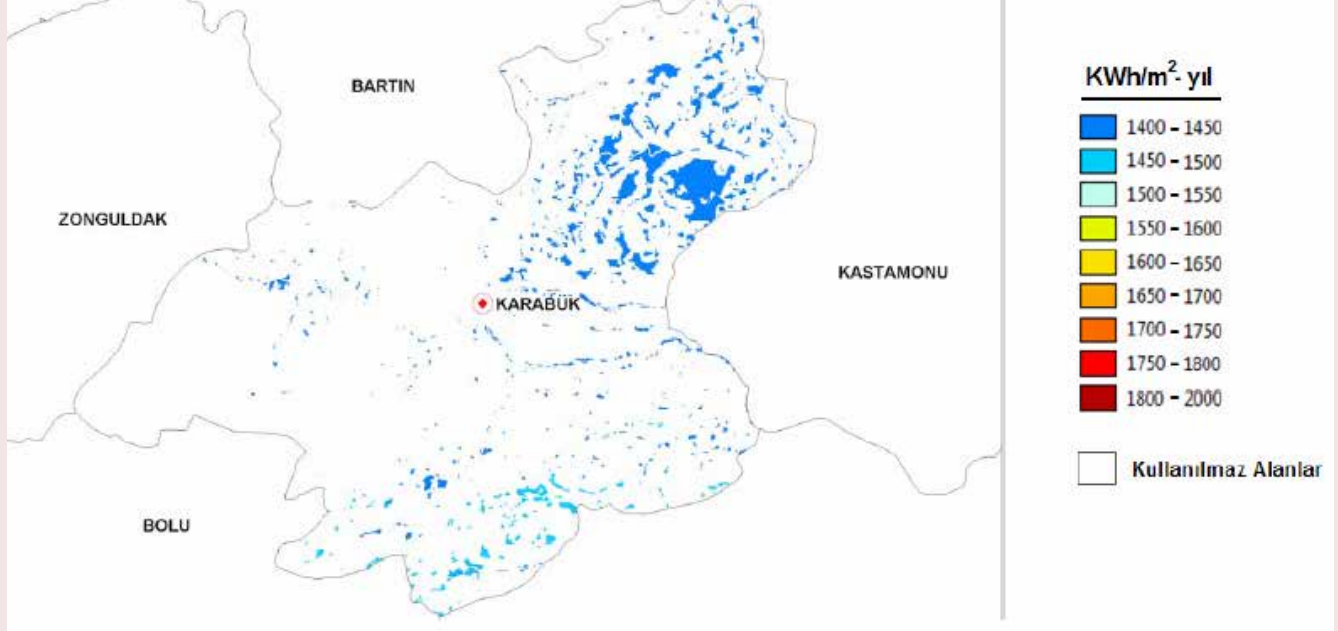
Şekil 3: Karabük ili güneş santrali potansiyeli
