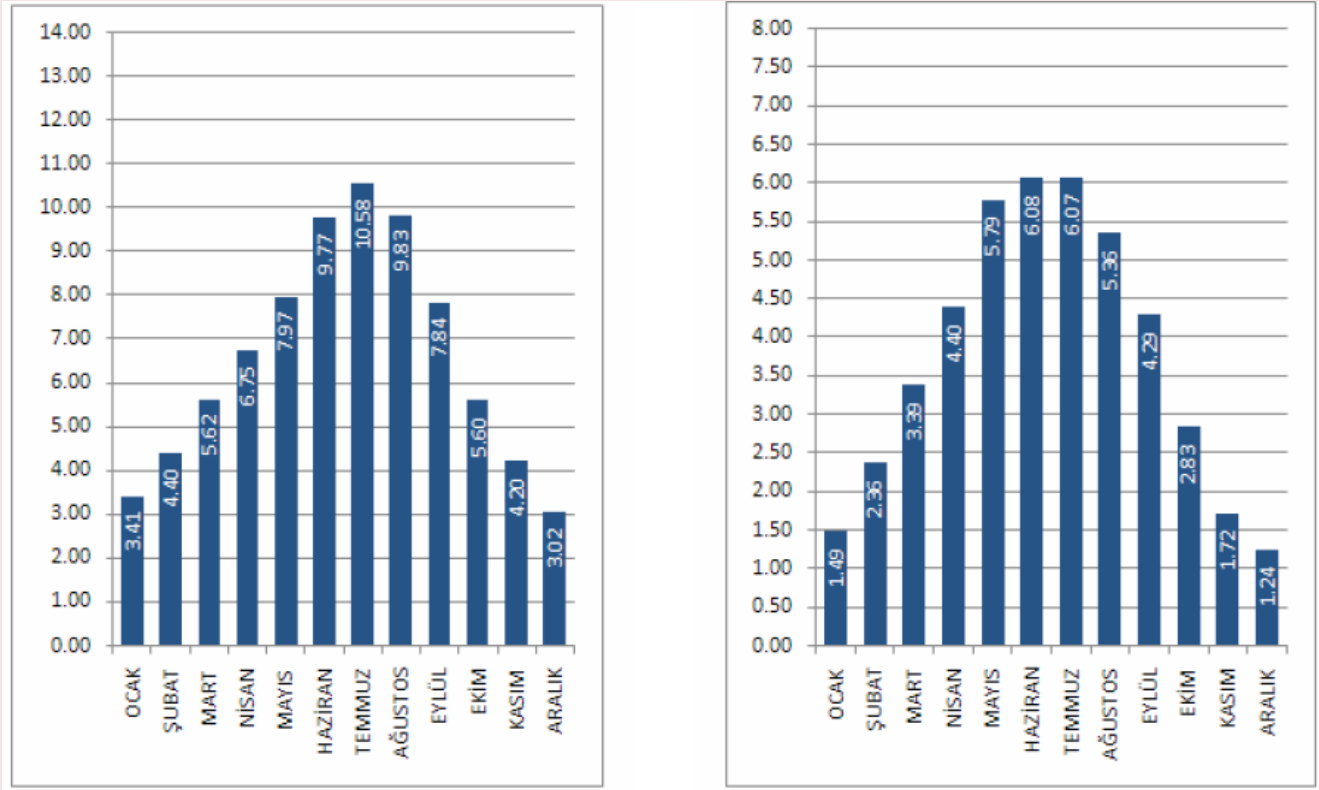
Şekil 1: Karabük ili güneşlenme süresi ve küresel radyasyon değerleri
