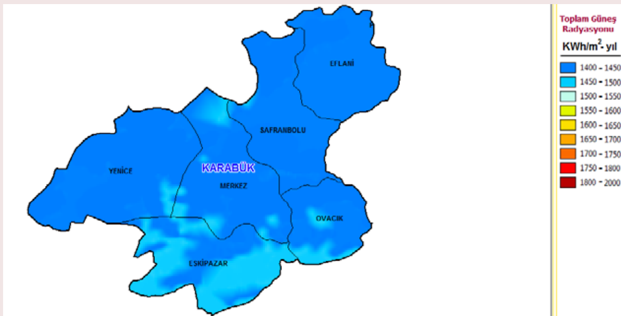
Şekil 2: Karabük ili küresel güneş radyasyon dağılımı
